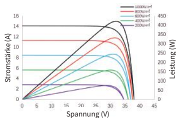
Strom/Leistungs-Spannungs-Kurve SSA-48HD-445N
