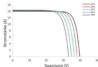
Strom-Spannungs-Kurve SSA-48HD-445N
